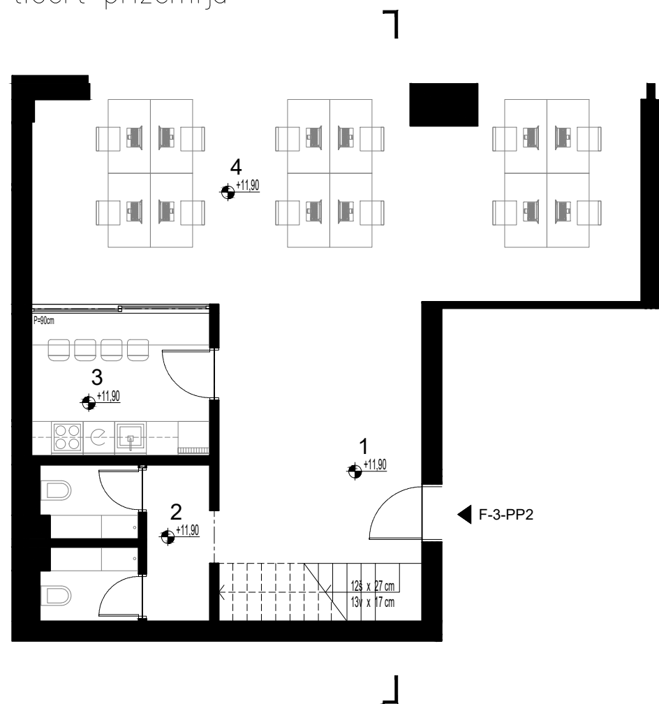
tlocrt prizemlja
