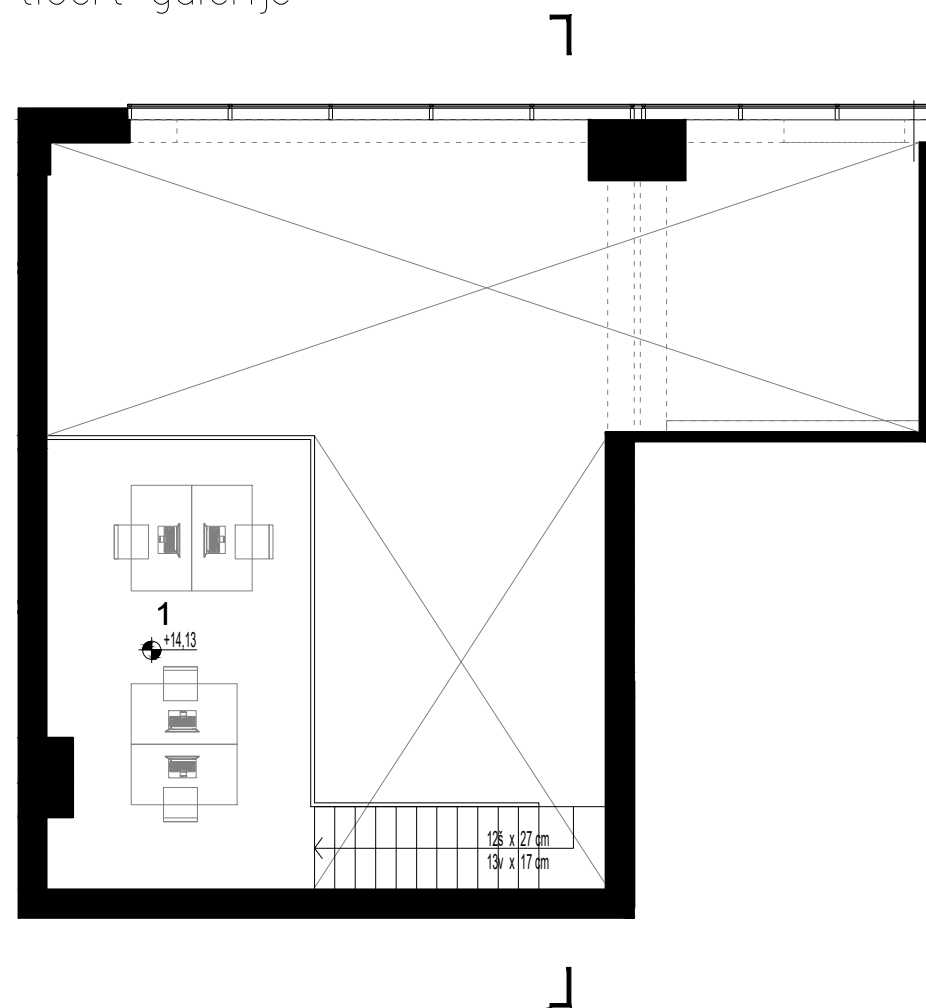
tlocrt galerije
