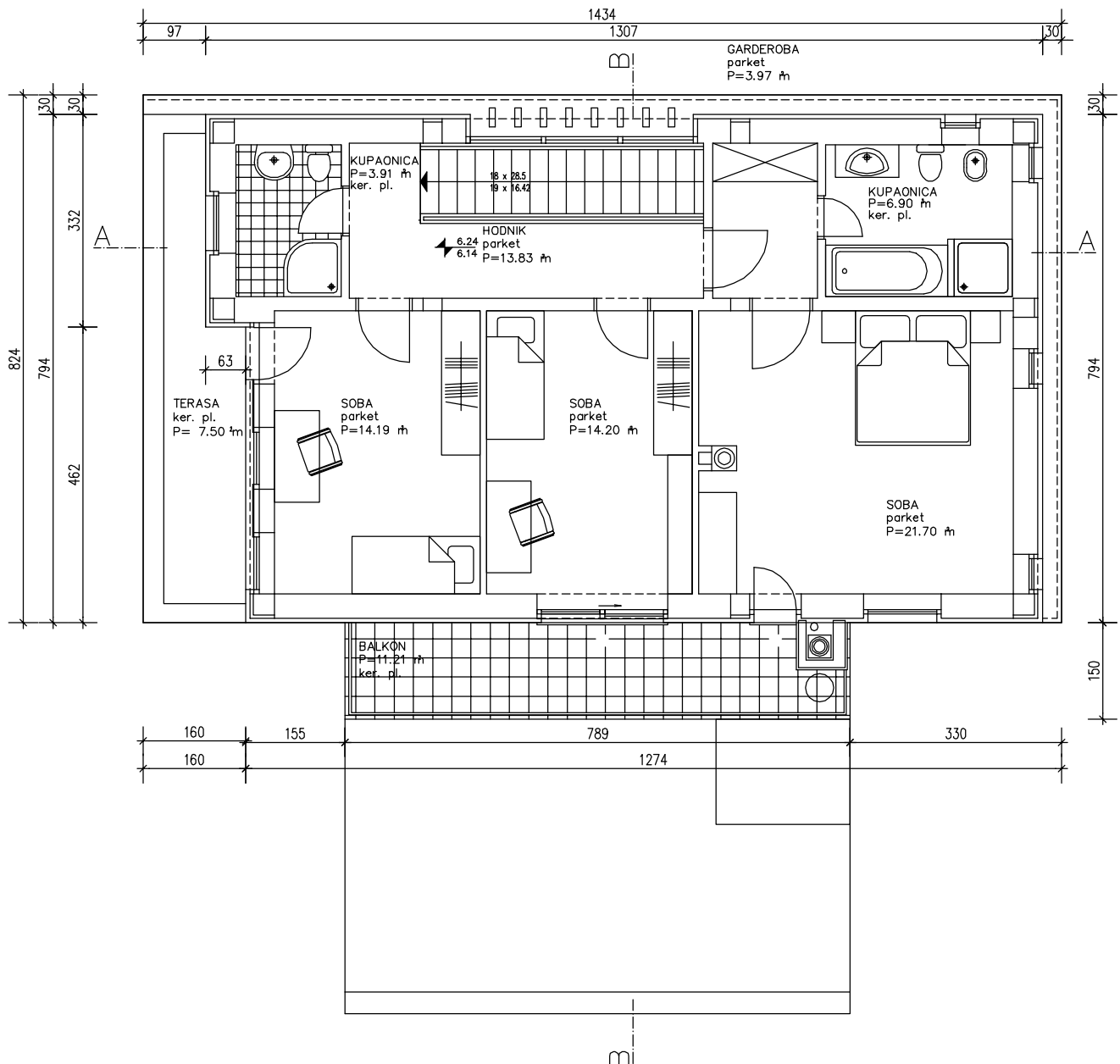
TLOCRT POTKROVLJA 1:100
